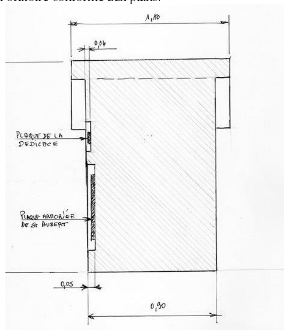
L'oratoire en coupe longitudinale
